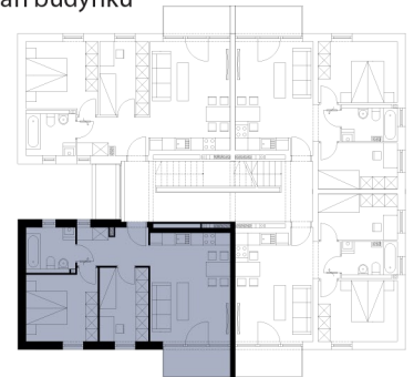
Plan budynku
